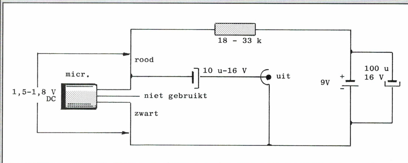
Fig. 5. De speciale voedingsschakeling om desgewenst een hogere signaalspanning (met toegenomen ruis, dat wel) te krijgen.
