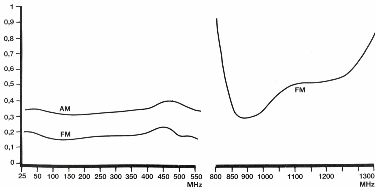
Fig. 1. Gevoeligheid Jupiteru MVT 6000 voor \text{dB } S+N/N verhouding.
